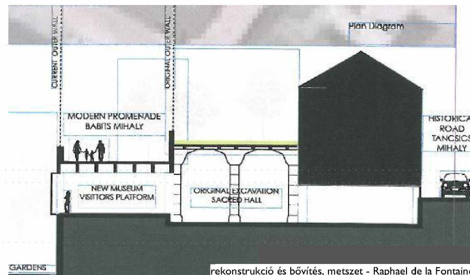
rekonstrukció és bővítés, metszet - Raphael de la Fontaine
