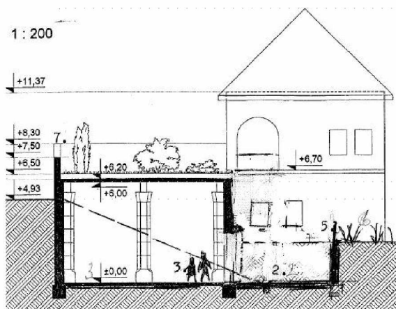
rekonstrukció síkfödémrel, metszet - Budai Aurél
