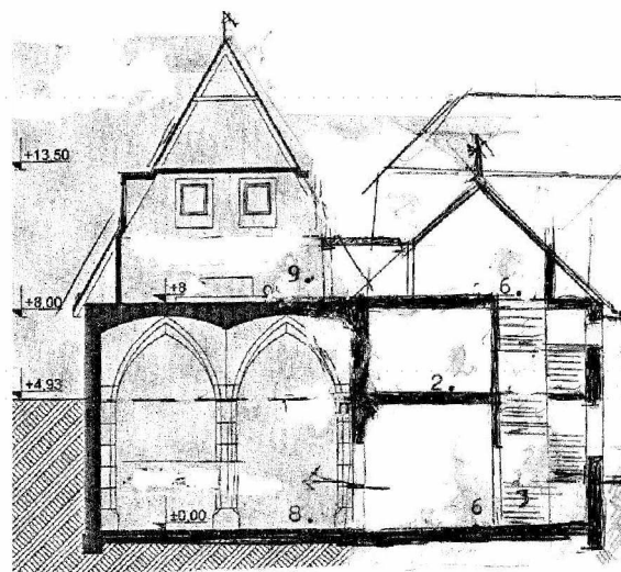
rekonstrukció boltozattal, metszet - Budai Aurél
